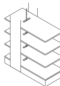
63/65 mm Lamellenbreite mit 38 mm Leiterband
