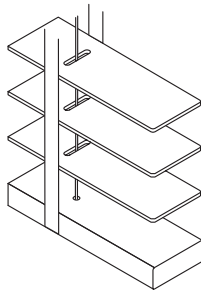
50 mm Lamellenbreite mit 10 mm Leiterband
