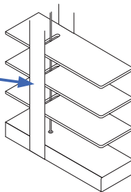
50 mm Lamellenbreite mit 24 mm Leiterband
