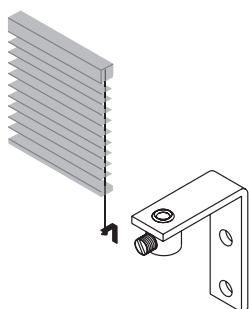
Vajerbeslag för väggmontage 25 & 50 mm lamellbredd Metallfärgat eller vitlackat
