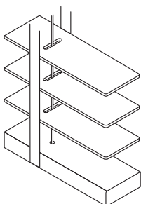
50 mm lamellbredd med 10 mm stegband
