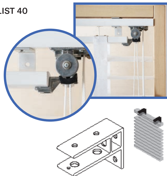
Universalbeslag till Överlist 40
